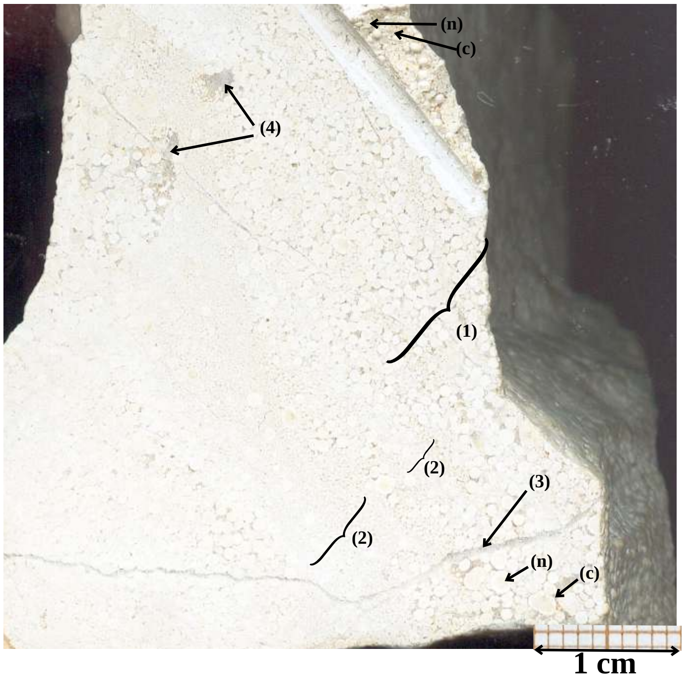
103_2 : Calcaire oolithique (x 4) montrant deux types de zone de dépôts
